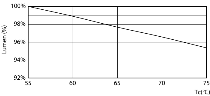
LEDtube COR 18W 30K LumenVsTc-LMP
