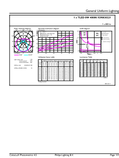
LEDtube COR 1 8W G13 800lm 840-GUL
